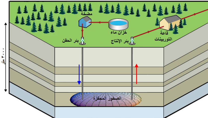
نظام الطاقة الجيوتحرارية المعززة النموذجي
